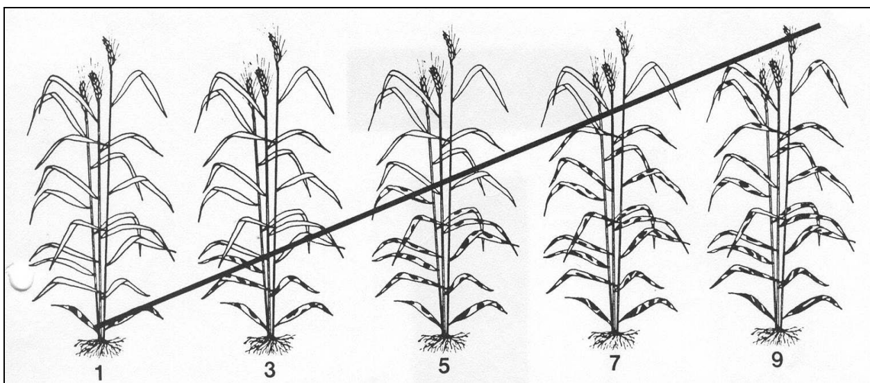
Saari-Prescott skála
