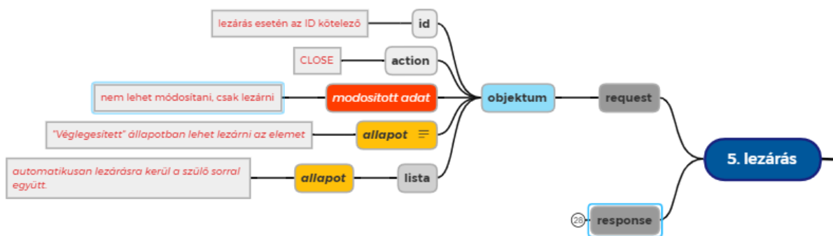
19. ábra – Adatsor lezárása – Request
