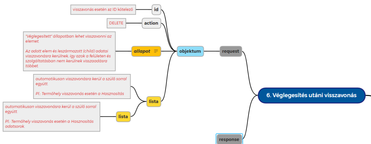
14. ábra – Adatsor törlése – Request és Response
