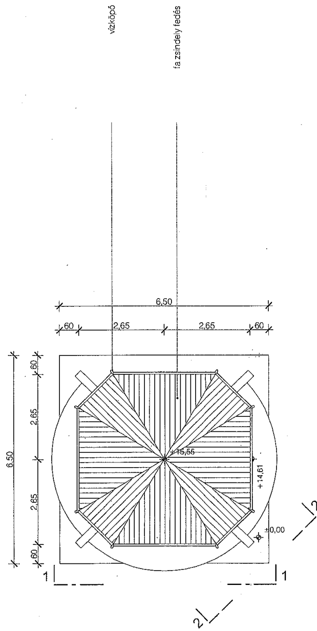
TETŐFELÜLNÉZET
