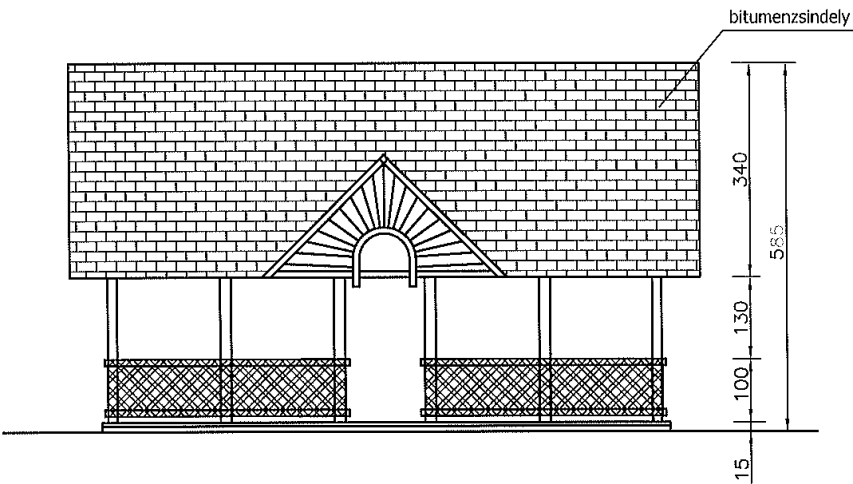
ELÖLNÉZET
