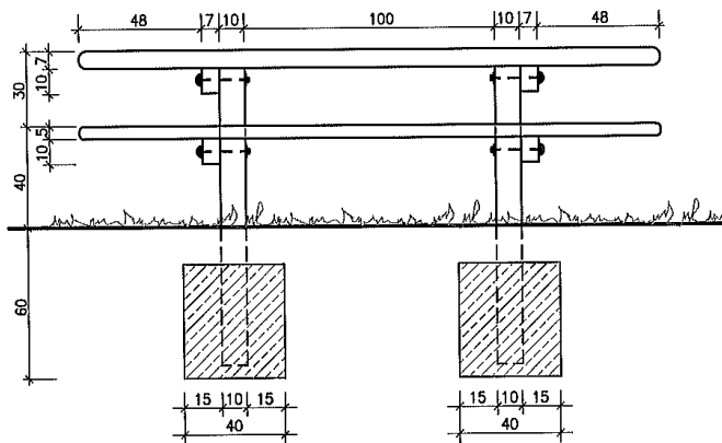
ELÖLNÉZET
