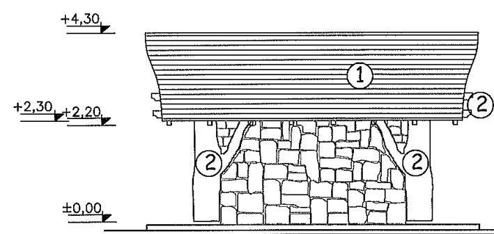
ELÖLNÉZET M = 1: 100
