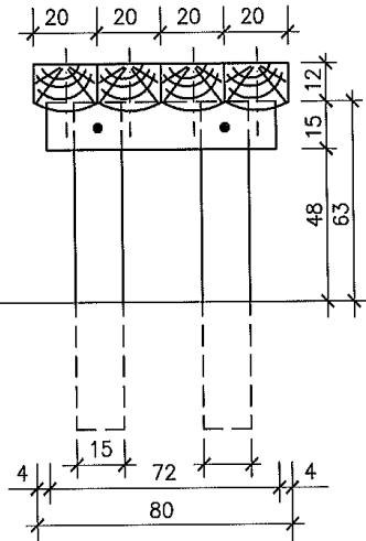
OLDALNÉZET
