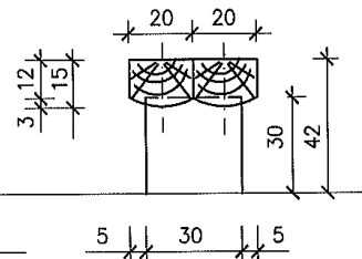
OLDALNÉZET
