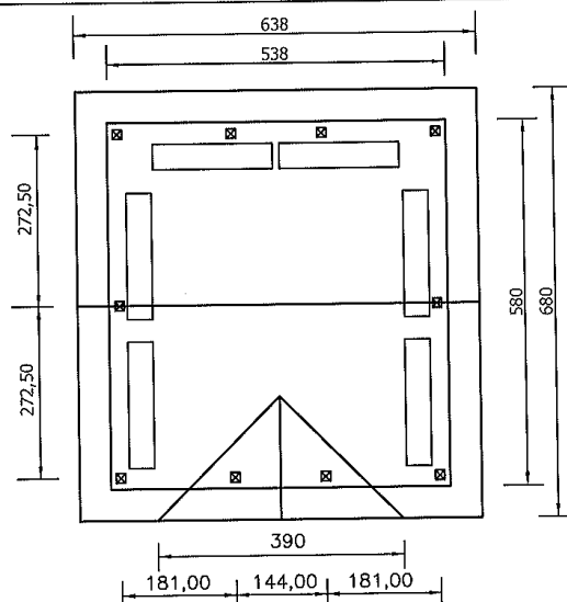
ALAPRAJZ
