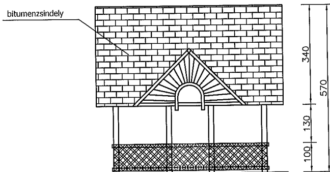
ELÖLNÉZET
