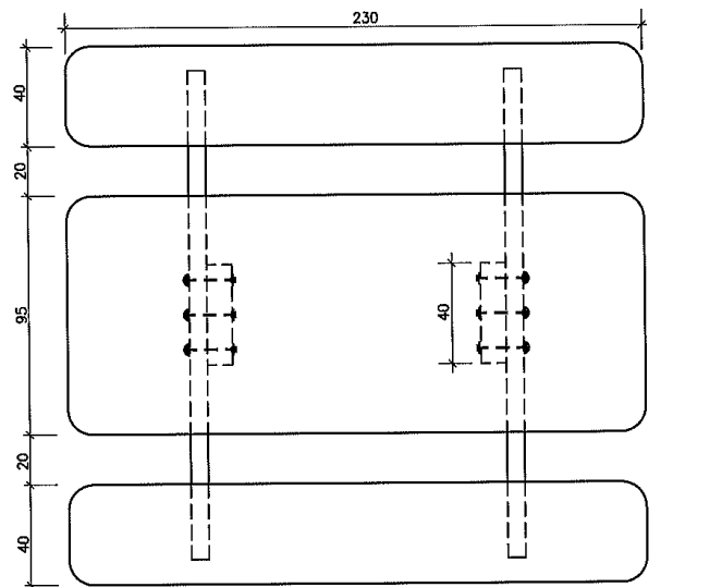
FELÜLNÉZET
