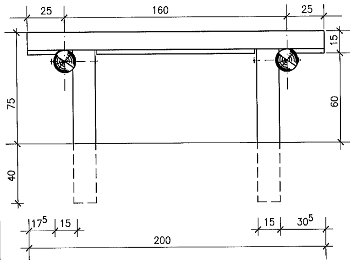
ASZTAL ELÖLNÉZET
