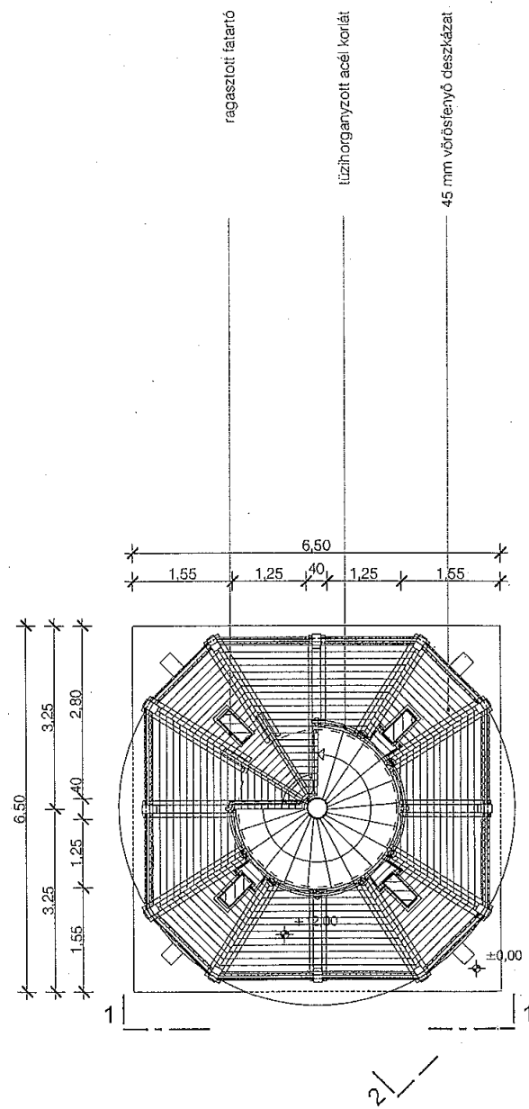
FELSŐ SZINTI ALAPRAJZ
