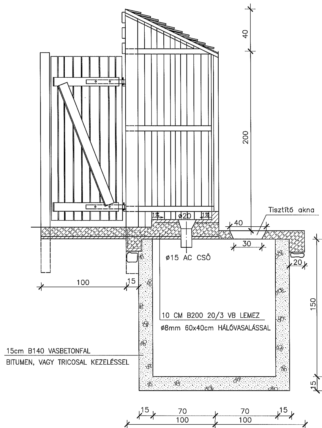
A - A METSZET
